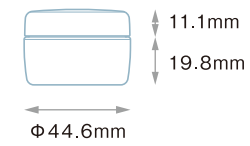
PCN-20 (PP) Rキャップ (PP)
