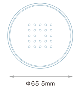
NFF-120FP 中蓋 (PE) 穴径：Φ2.0mm
