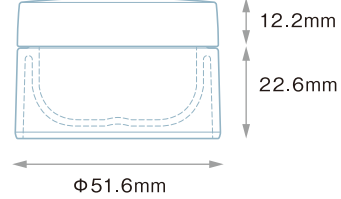
ANC-30 (PP) Fキャップ(PP)
