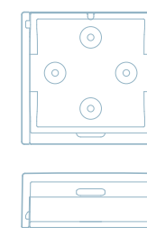
Assort S ケース (AS/ABS) ※Sコマのみセット可能
