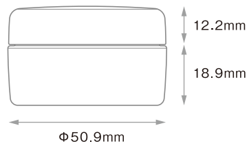
PCN-30(PP) Rキャップ(PP)
