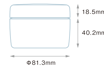
PCN-180 (PP) Rキャップ (PP)
