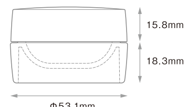
PCL-20(PP) キャップ(PP)
