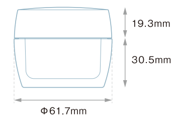
PCI-60 (PP/PP) キャップ (PP)
