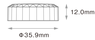
PCL-5 Tキャップ(PP)
