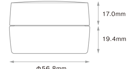
PCL-30(PP) キャップ(PP)
