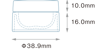
ANC-10 (PP) Fキャップ(PP)
