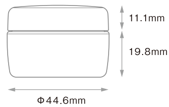
PCN-20(PP) Rキャップ(PP)
