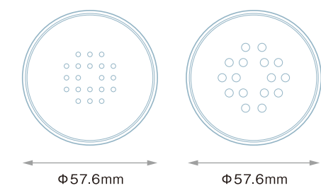
APN パウダー中蓋 (PE) 穴径：Φ2.0・Φ3.5mm
