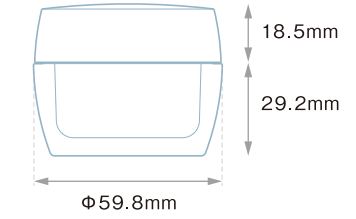
PCI-50 (PP/PP) キャップ (PP)
