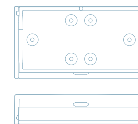
Assort M ケース (AS/ABS) ※Mコマのみセット可能
