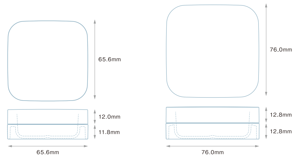
ガレット Galette-30 (PP) キャップ (PP) O.F.容量 : 33.8ml
