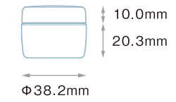
PCN-15 (PP) Rキャップ (PP)
