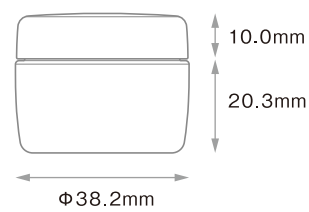
PCN-15(PP) Rキャップ(PP)
