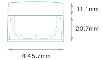
ANC-20 (PP) Fキャップ(PP)
