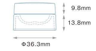
ANC-5 (PP) Fキャップ(PP)
