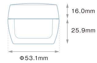
PCI-30 (PP/PP) キャップ (PP)
