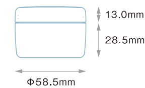
PCN-60 (PP) Rキャップ (PP)
