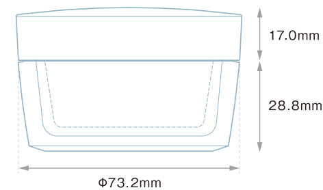
CPA-50 (AS/PP) キャップ (ABS) O.F.容量 : 70.0ml
