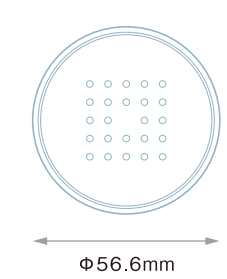
NFF-80FP 中蓋 (PE) 穴径：Φ2.0mm
