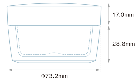
CPA-60 (AS/PP) キャップ (ABS) O.F.容量 : 80.6ml
