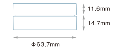
APN パウダー (AS) キャップ (AS) 容量：約7~8g
