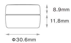
PCN-3(PP) Rキャップ(PP)
