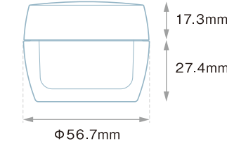
PCI-40 (PP/PP) キャップ (PP)
