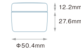
PCN-40 (PP) Rキャップ (PP)
