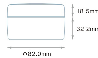
PCN-150 (PP) Rキャップ (PP)
