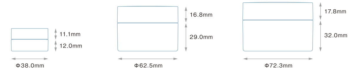
NFF-10FP (AS) キャップ (ABS) 容量：約2~3g
