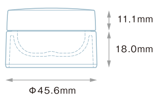
ANC-15 (PP) Fキャップ(PP)
